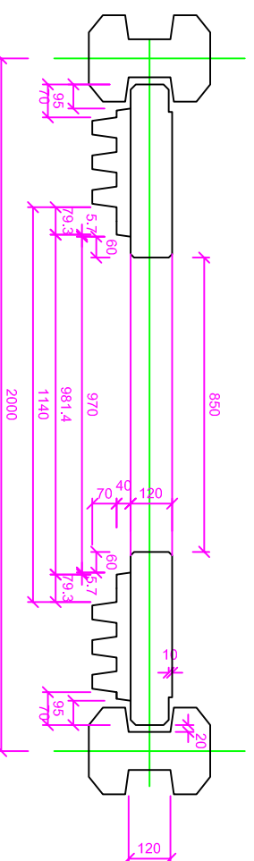
PRZEKRÓJ B - B
