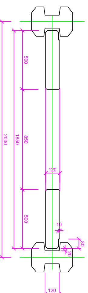
PRZEKRÓJ B - B
